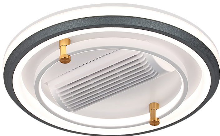
ITEM NO : 3319R LAMP SIZE:500*500*150mm CCT:Dimming 3000-6500K MAT. : IRON+ACRYLIC ACTUAL WATT. : LED62W
