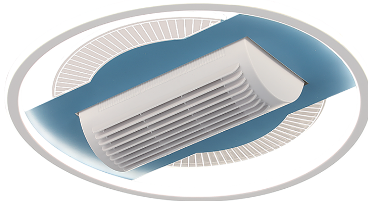
ITEM NO : 1349-3 LAMP SIZE:500*150mm CCT:Dimming 3000-6500K MAT. : IRON+ACRYLIC ACTUAL WATT. : LED45W
